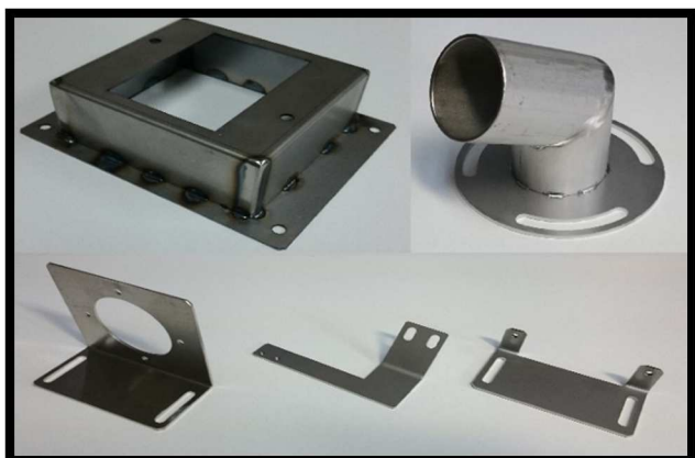
板金加工例
