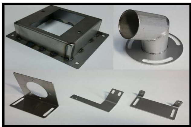
板金加工例
